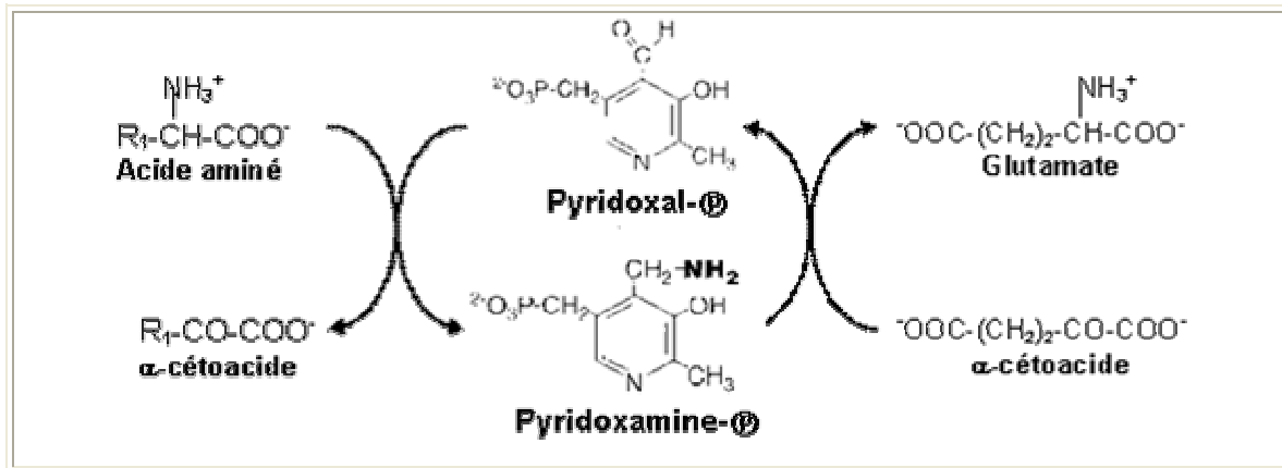
Figure 1 - Schéma général de la réaction catalysée par une aminotransférase.
