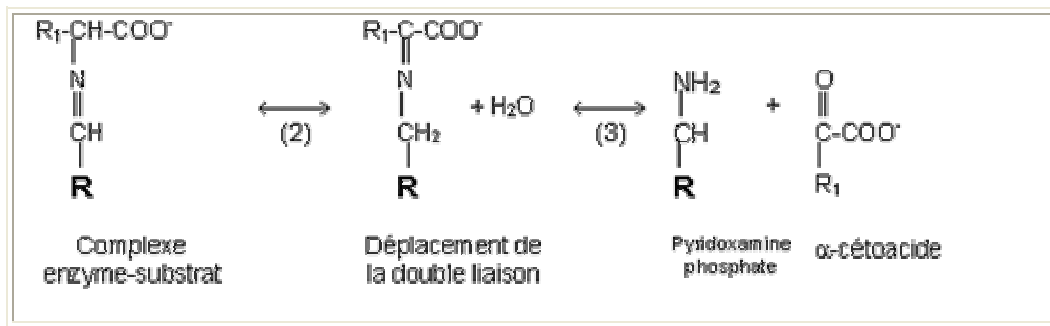
Figure 2 - Mécanisme de la transamination : (1) Prise en charge de l'acide aminé avec ormatie liaison covalente (imine = base de Schiff) ; (2) Déplacement de la double liaison ; (3) Hydrolyse
