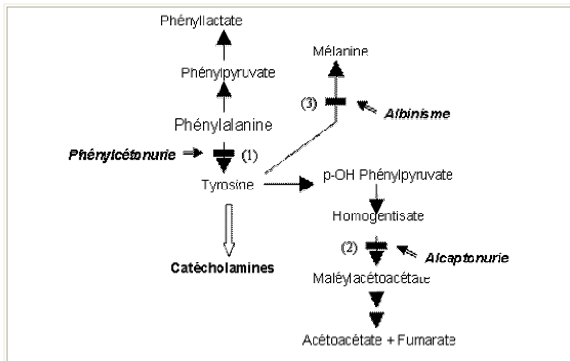
Figure 6 – Résumé du catabolisme de la phénylalanine et de la tyrosine. Des déficiences enzymatiques de phénylalanine oxydase au niveau (1) provoque la phénylcétonurie – de homogentisate oxydase au niveau (2) l'alcaptonurie – d'une enzyme au niveau (3) l'albinisme.
